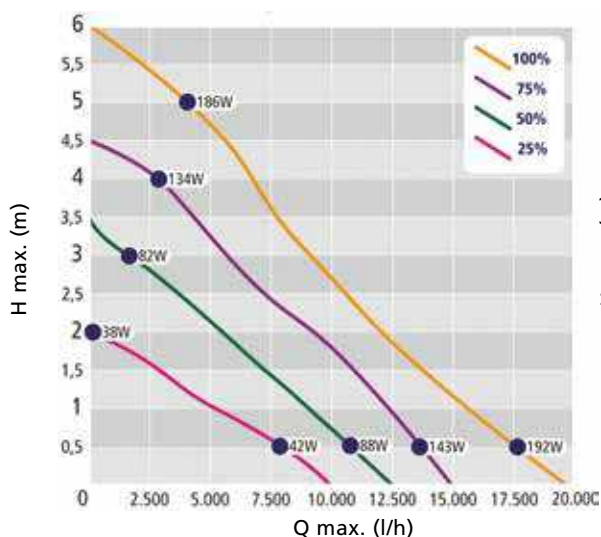
Pompgrafiek VarioFlow® 20
