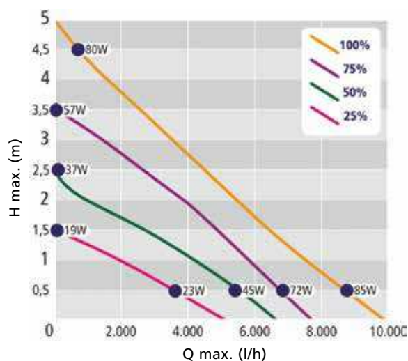
Pompgrafiek VarioFlow® 10
