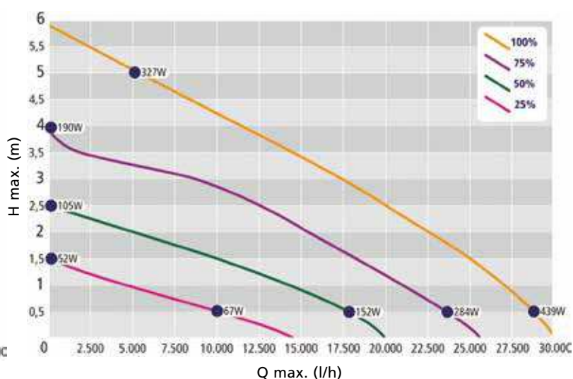
Pompgrafiek VarioFlow® 30
