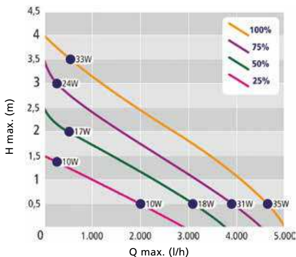
Pompgrafiek VarioFlow® 5
